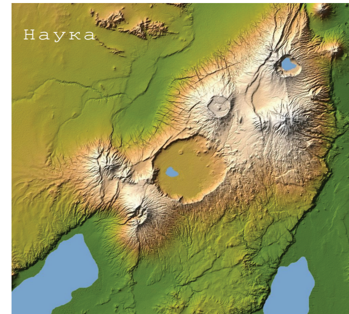
Рис. 6. Кальдера Нгоронгоро
