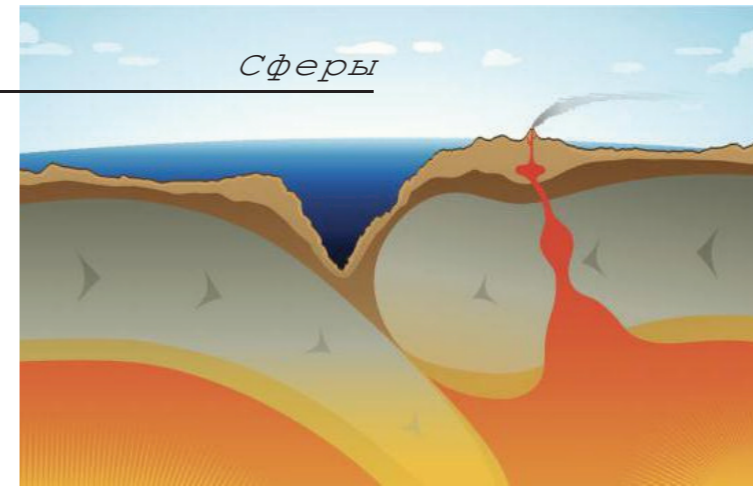
Рис. 1. Процесс вулканообразования
